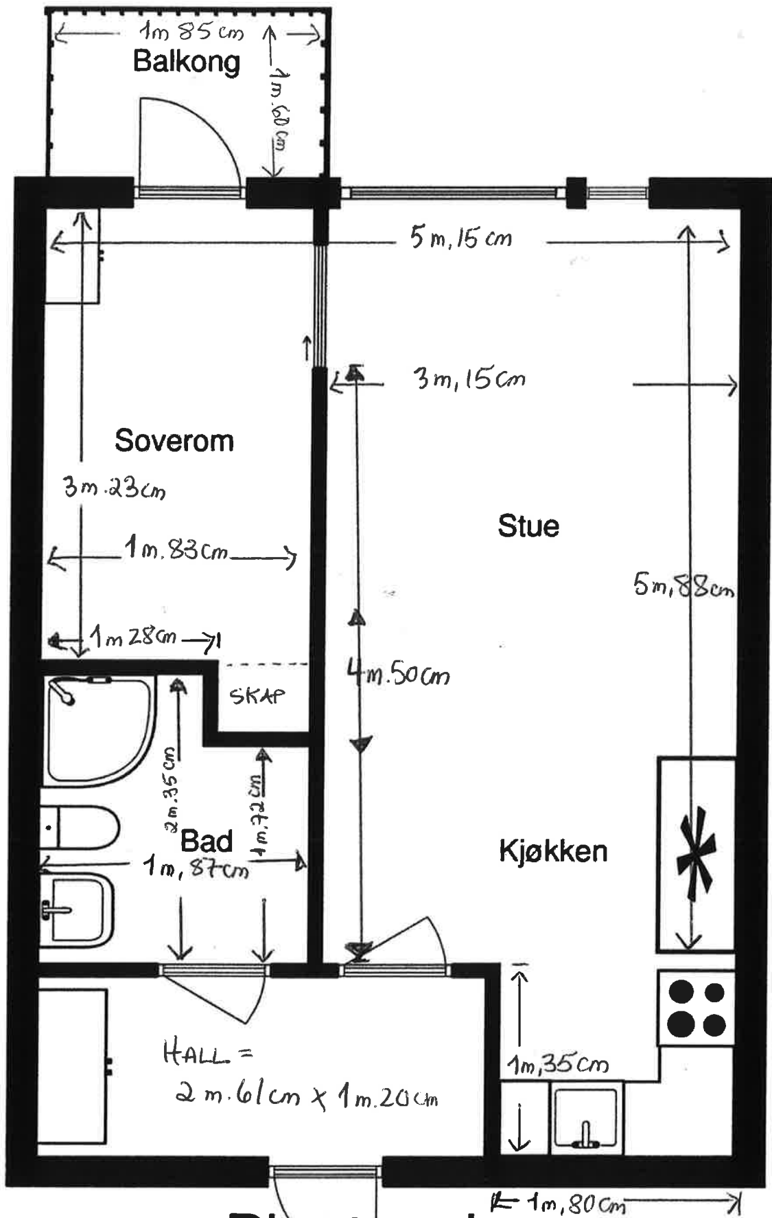
Plantegning
